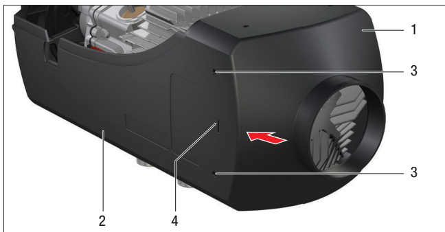
1 Utloppshuv 2 Mantelkåpa undre 3 Snäpplås 4 Ursparning
