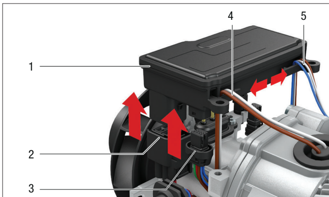
1 Styrdon 3 Kontakt kabelstam 2 Kontakt strömförsörjning och glödstift 4 Anslutning glödstift 5 Anslutning kombisensor
