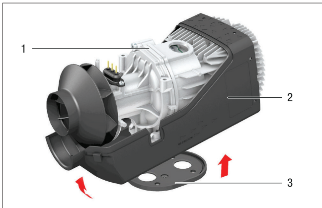
1 Värmare 2 Mantelkåpa undre 3 Flänstätning
