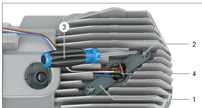
1 Monteringsfästen 3 Flatskruvmejsel 2 Klor 4 Kombisensor
