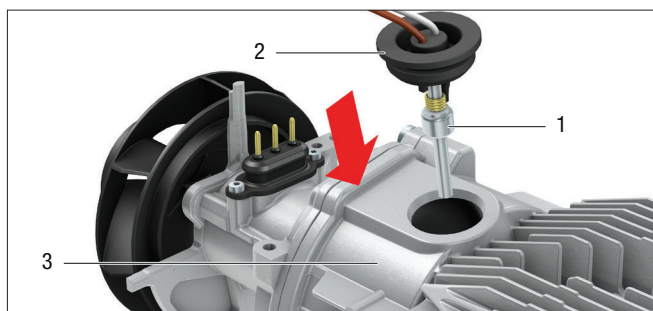
1 Glödstift 3 Värmeväxlare 2 Gummibussning
