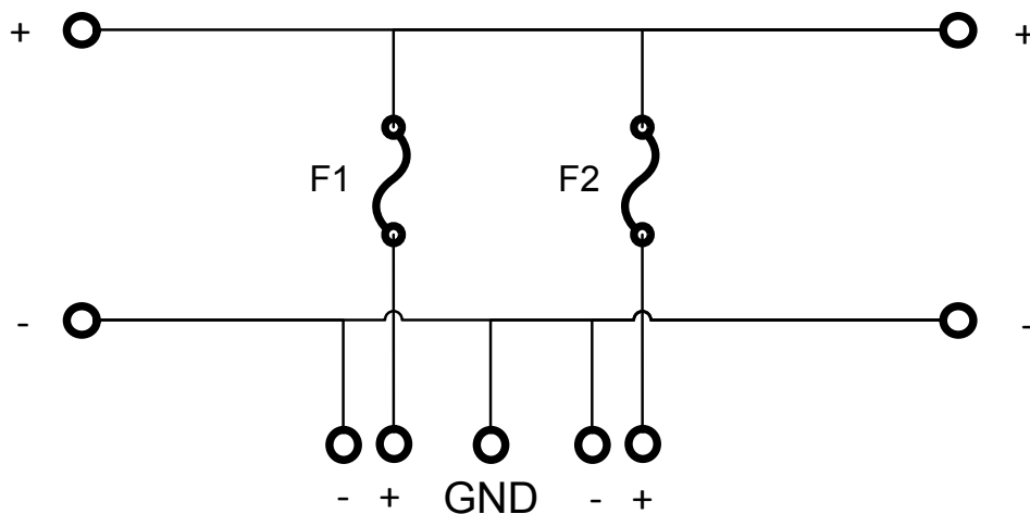
Det interna kopplingsschemat för Lynx Class-T Power In
