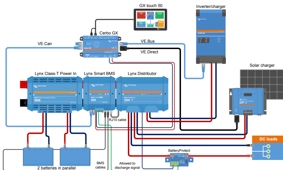
System med Lynx Class-T Power In, två smarta litiumbatterier, ett Lynx Smart BMS och en Lynx Distributor
