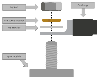
Figur 3. Korrekt monteringssekvens av DC-kablar.
