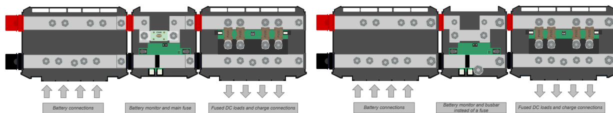
Sammankopplade Lynx-moduler: Lynx Power In, Lynx Shunt VE.Can och Lynx Distributor. Till höger finns M10-varianten med samlingskena istället för säkringen.
