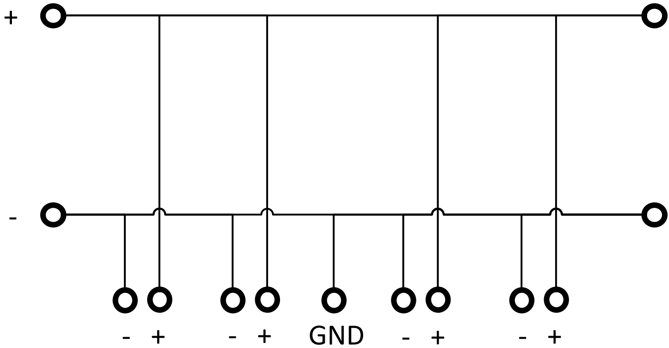
Kopplingsschemat för Lynx Power In
