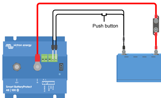
Tryckknapp kopplad för att programmera Smart BatteryProtect
