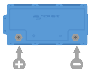
Batteriterminaler
