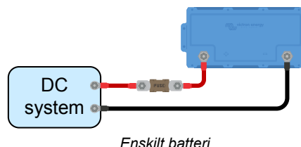
Enskilt batteri
