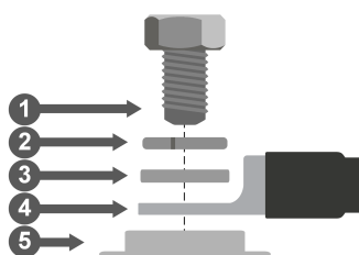
Koppling av batterikablar
