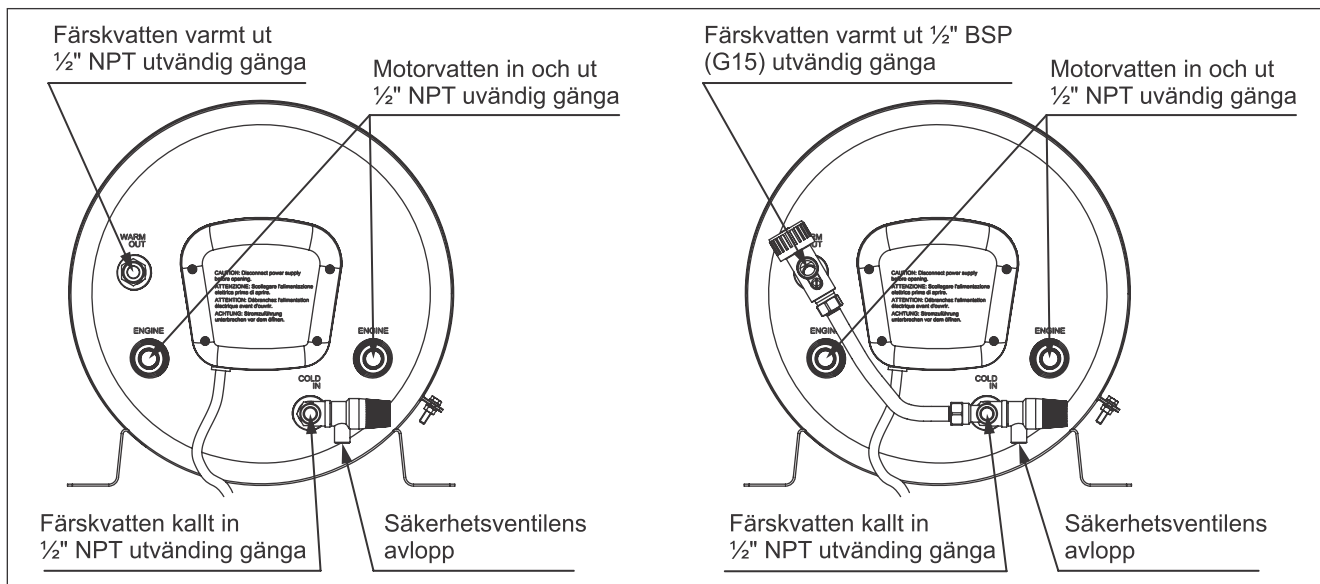
Fig. 4 Observera: Slangnipplar med rak 1/2" BSP gänga passar även till 1/2" NPT utvändig gänga.
