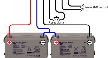
Balanseringsenhet (BMS012201000) Balanseringsenheten utjämnar laddningstillståndet hos två seriekopplade 12 V batterier eller hos flera rader av seriekopplade batterier. När laddningsspänningen för ett 24 V batterisystem ökar till mer än 24 V kommer balanseringsenheten att slå på och jämföra spänningen över de två seriekopplade batterierna. Balanseringsenheten kommer att dra en ström på upp till 1 A från batteriet (eller de parallellkopplade batterierna) med den högsta spänningen. Den resulterande laddningsströmmen kommer att säkerställa att batterierna kommer att nå samma laddningstillstånd.
