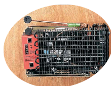
"KLICK"! Där sitter kompressorn, låst utan några verktyg eller passningar.
