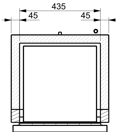
SEZIONE B-B
